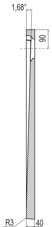
COUPE B-B
