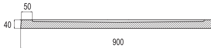
COUPE C-C
